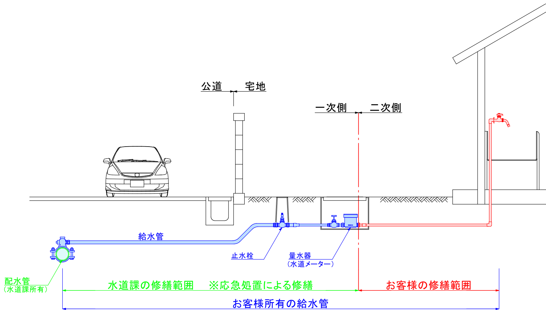
直結直圧方式の場合
