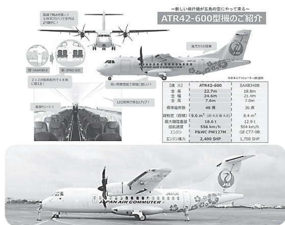
来年度から就航するATR機48人乗り
