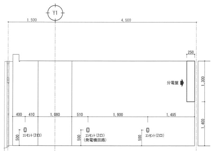
展開図 D面
