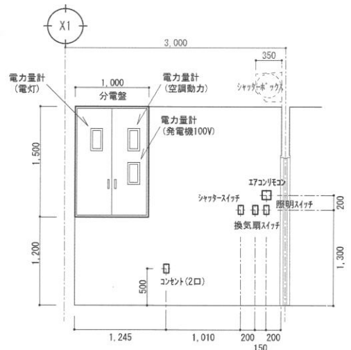
展開図 A面
