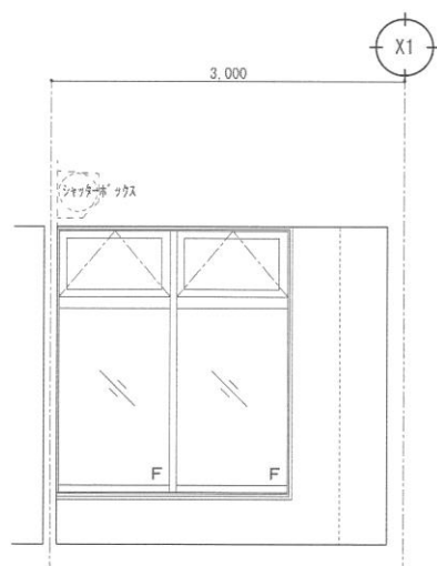
展開図 C面
