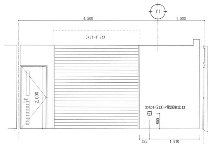
展開図 B面
